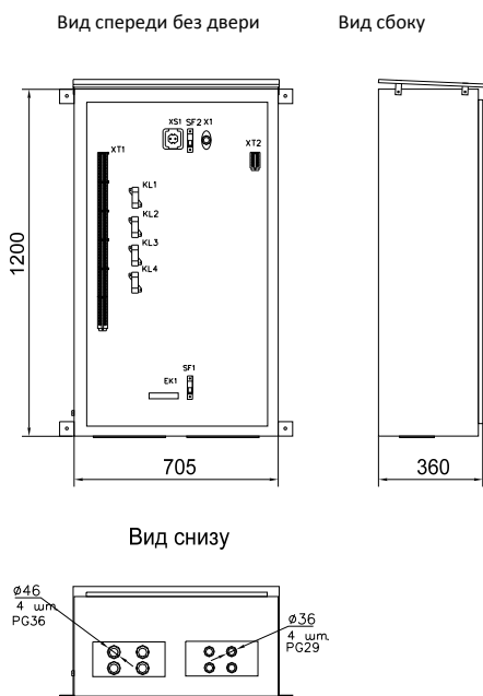
Рис. 8.6.1. Внешний вид шкафа ШРП-4.
