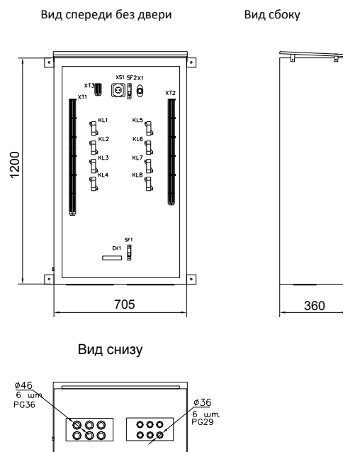
Рис. 8.6.2. Внешний вид шкафа ШРП-8.
